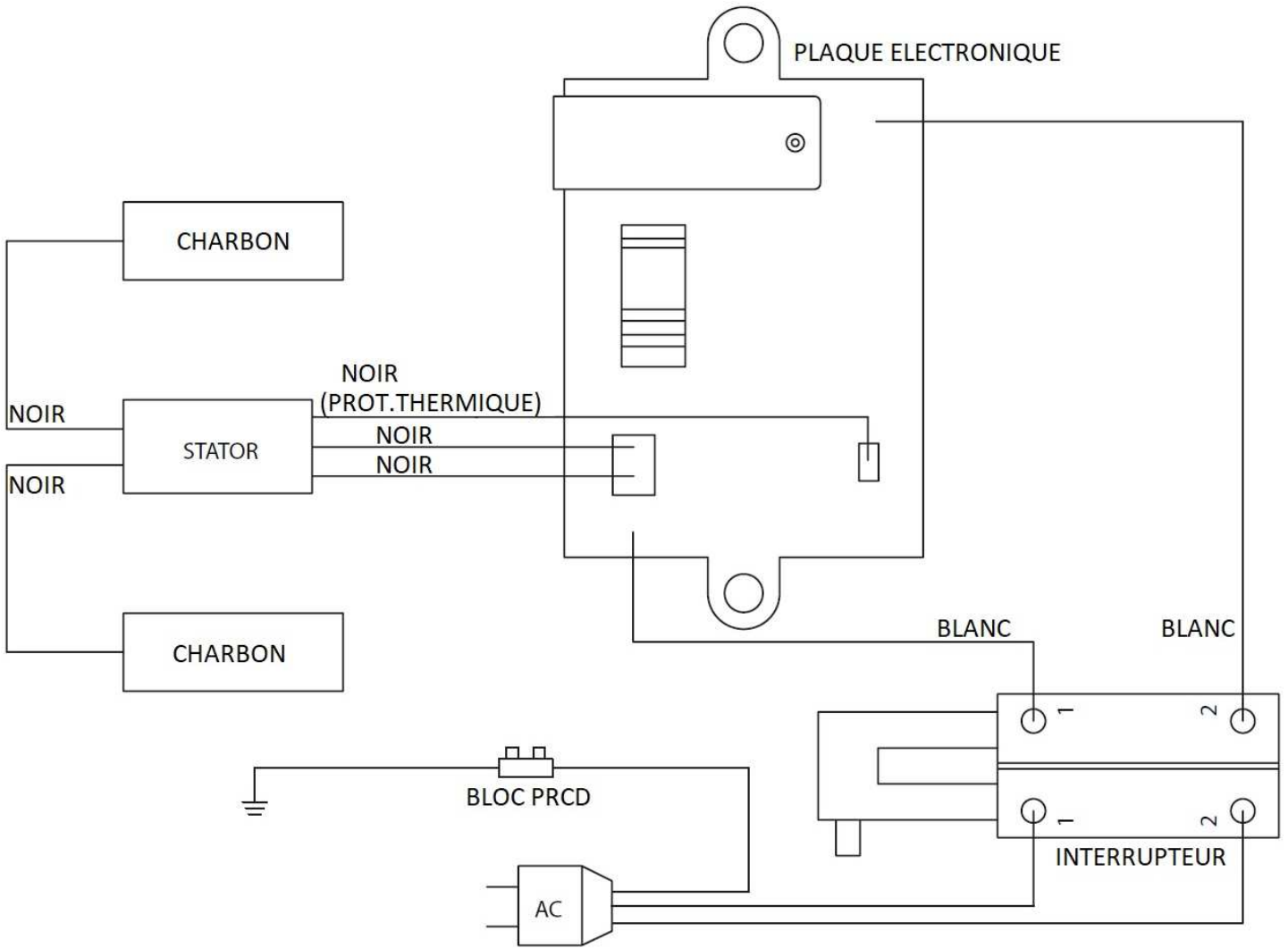
SCHEMA ELECTRIQUE PRO CD 182-S
