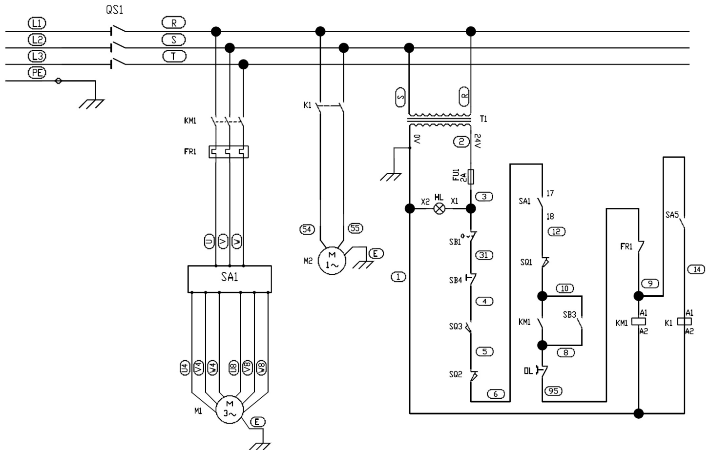
NOMENCLATURE SCHEMA ELECTRIQUE EXPERT 250 SR DA TRI (VUE 06)
