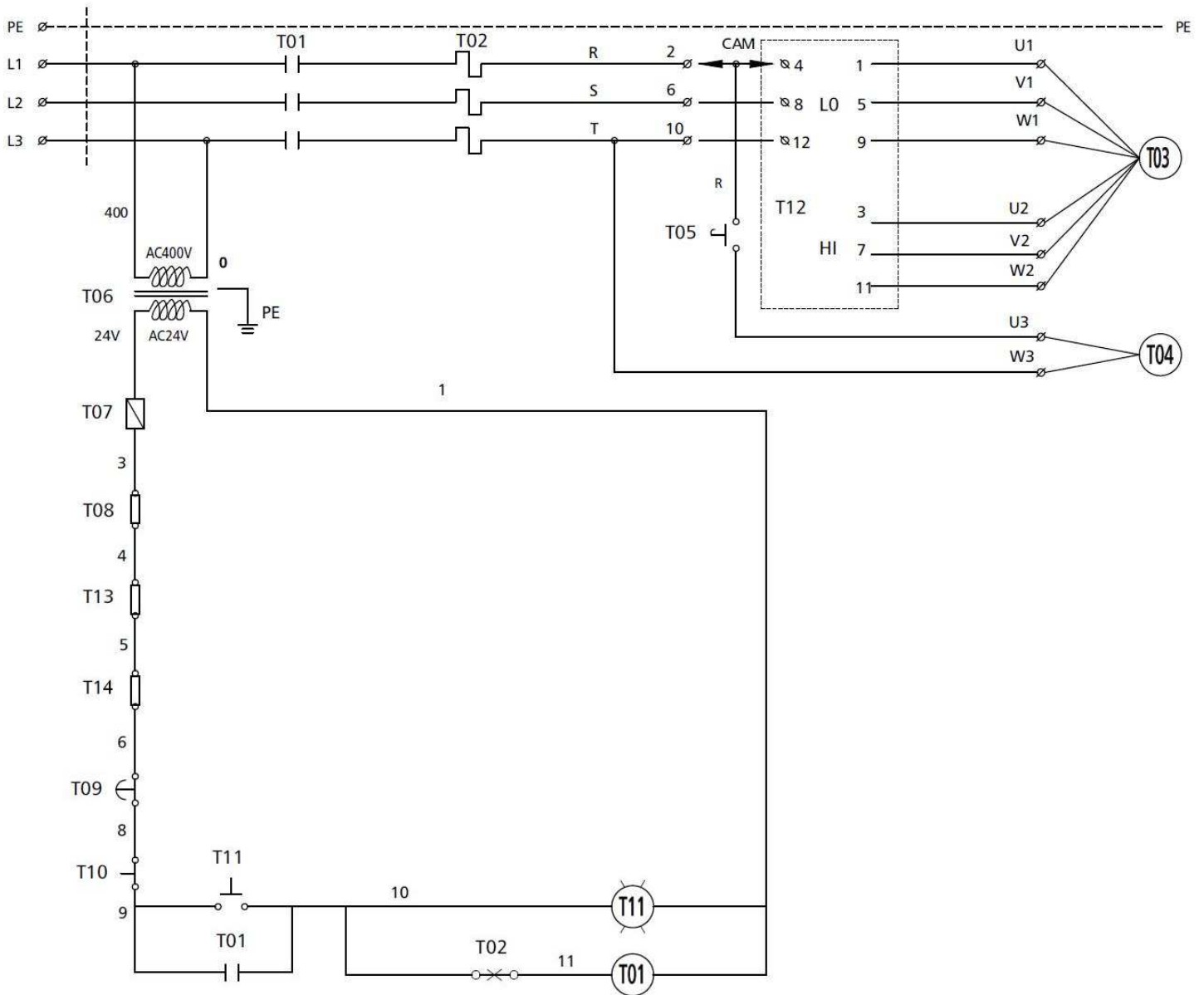
SCHEMA ELECTRIQUE SR276DA tri (VUE 02)
