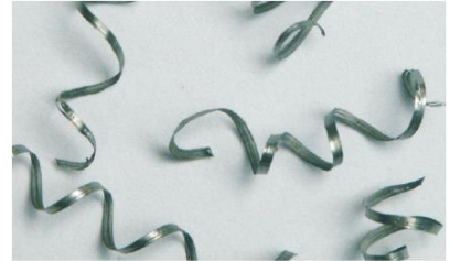
L'enroulement modéré des copeaux indique des conditions de coupe correctes
