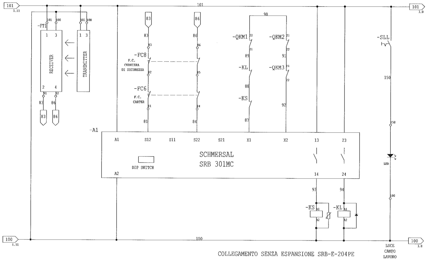
SCHEMA ELECTRIQUE SR260BAV (VUE 11)
